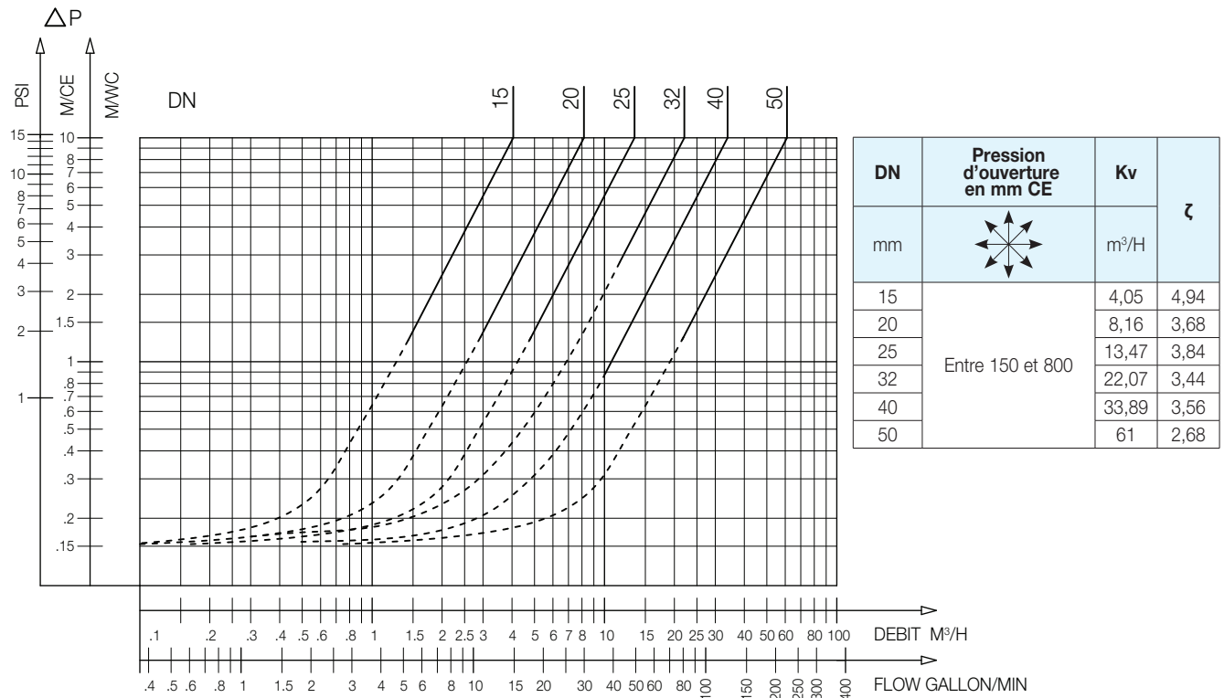
EA 223D - Abaque des pertes de charge
