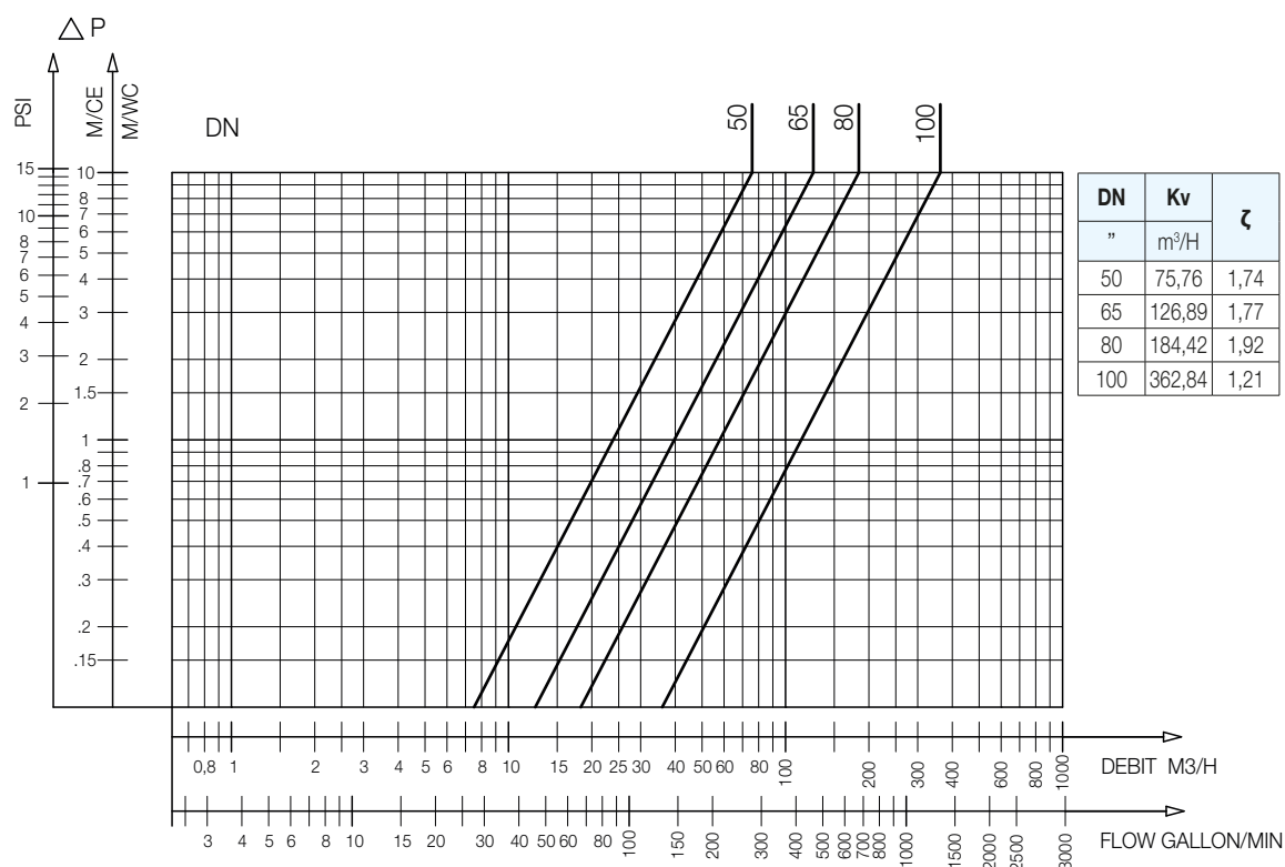
46 - Abaque des pertes de charge
